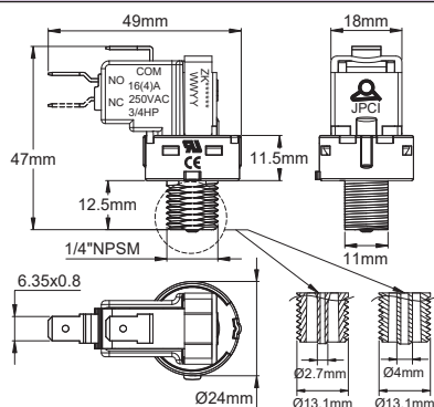
Filetage 1/4" NPSM
